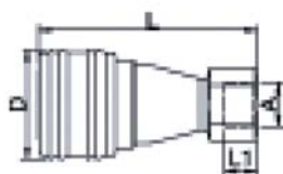
Kupplung
