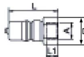
Nippel
